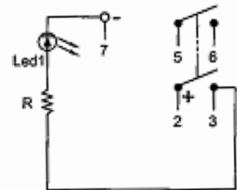
5P DPST OFF-ON (LED-D)
