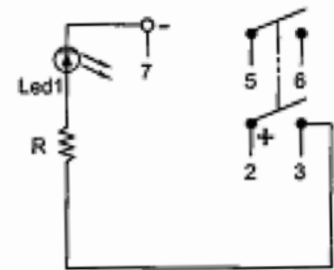
5P DPST OFF-ON (LED-D)
