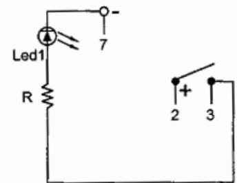
3P SPST OFF-ON (LED-D)
